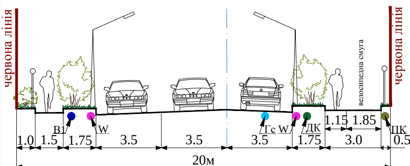
ПРОФІЛЬ 1-1
