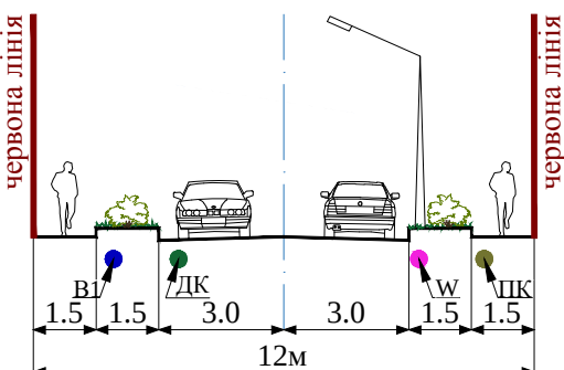
ПРОФІЛЬ 3-3
