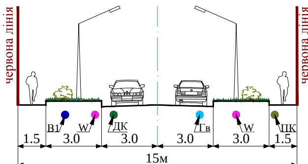
ПРОФІЛЬ 2-2
