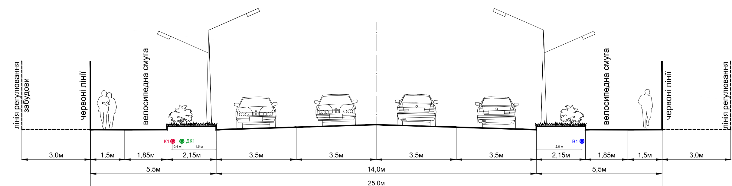
ПРОФІЛЬ І-І
