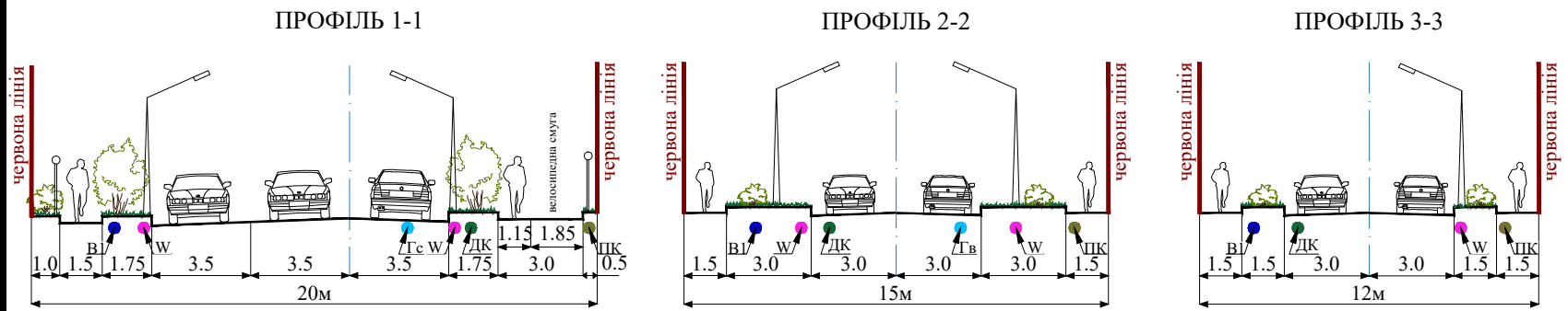
ПОПЕРЕЧНІ ПРОФІЛІ ВУЛИЦЬ: (М 1:200)
