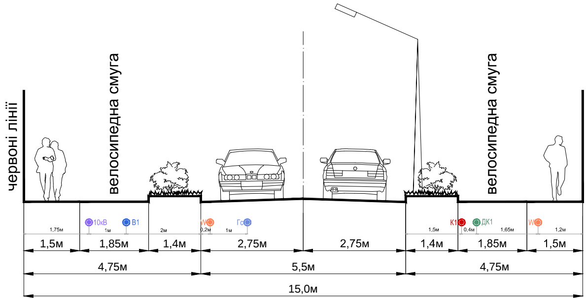
ПРОФІЛЬ ІІІ-ІІІ
