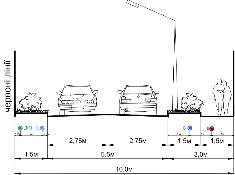
ПРОФІЛЬ ІІ-ІІ
