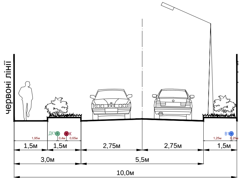
ПРОФІЛЬ ІІІ-ІІІ
