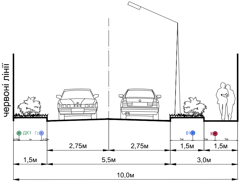
ПРОФІЛЬ ІІ-ІІ
