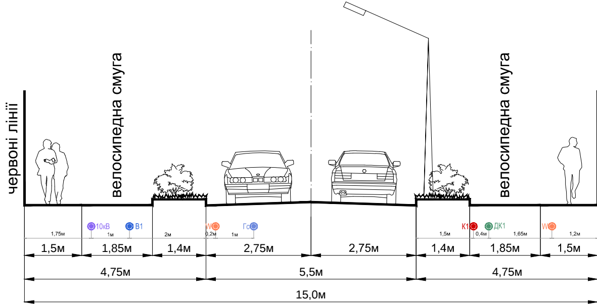
ПРОФІЛЬ ІІІ-ІІІ
