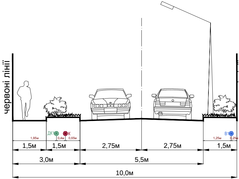
ПРОФІЛЬ І-І
