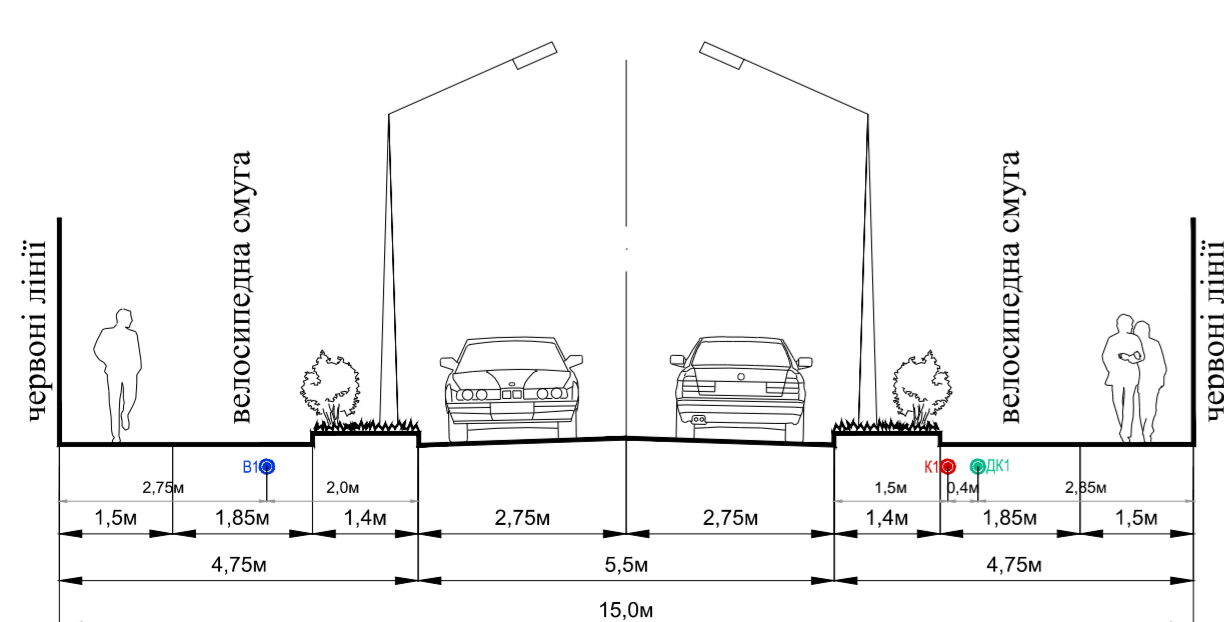
ПРОФІЛЬ І-І
