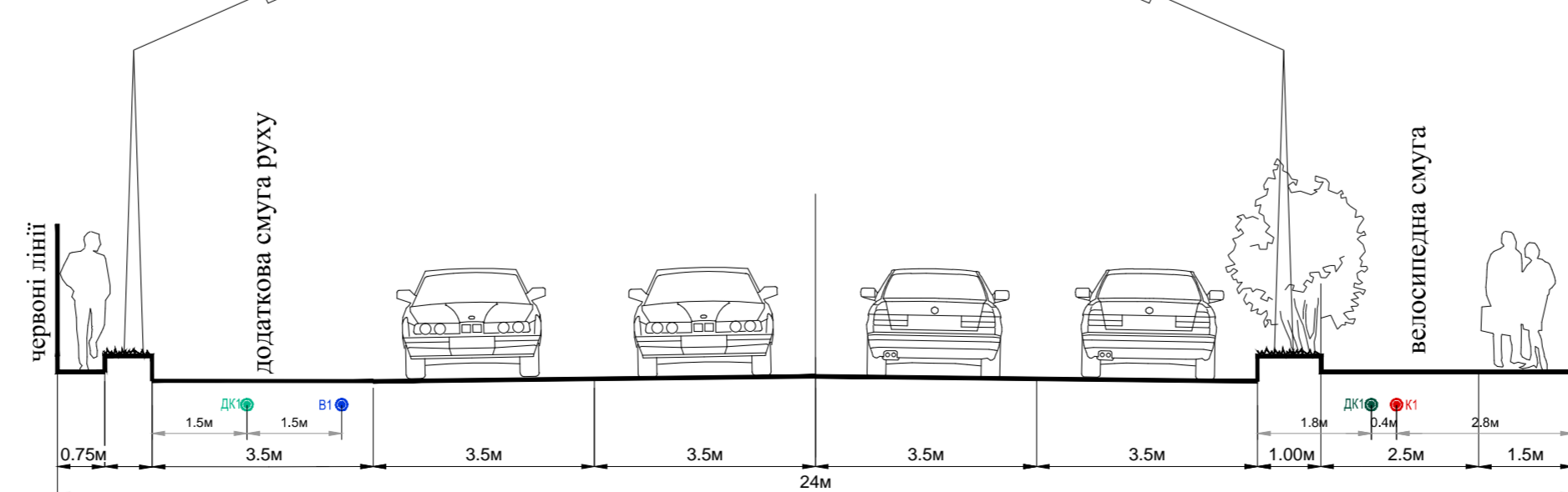
ПРОФІЛЬ ІІ-ІІ
