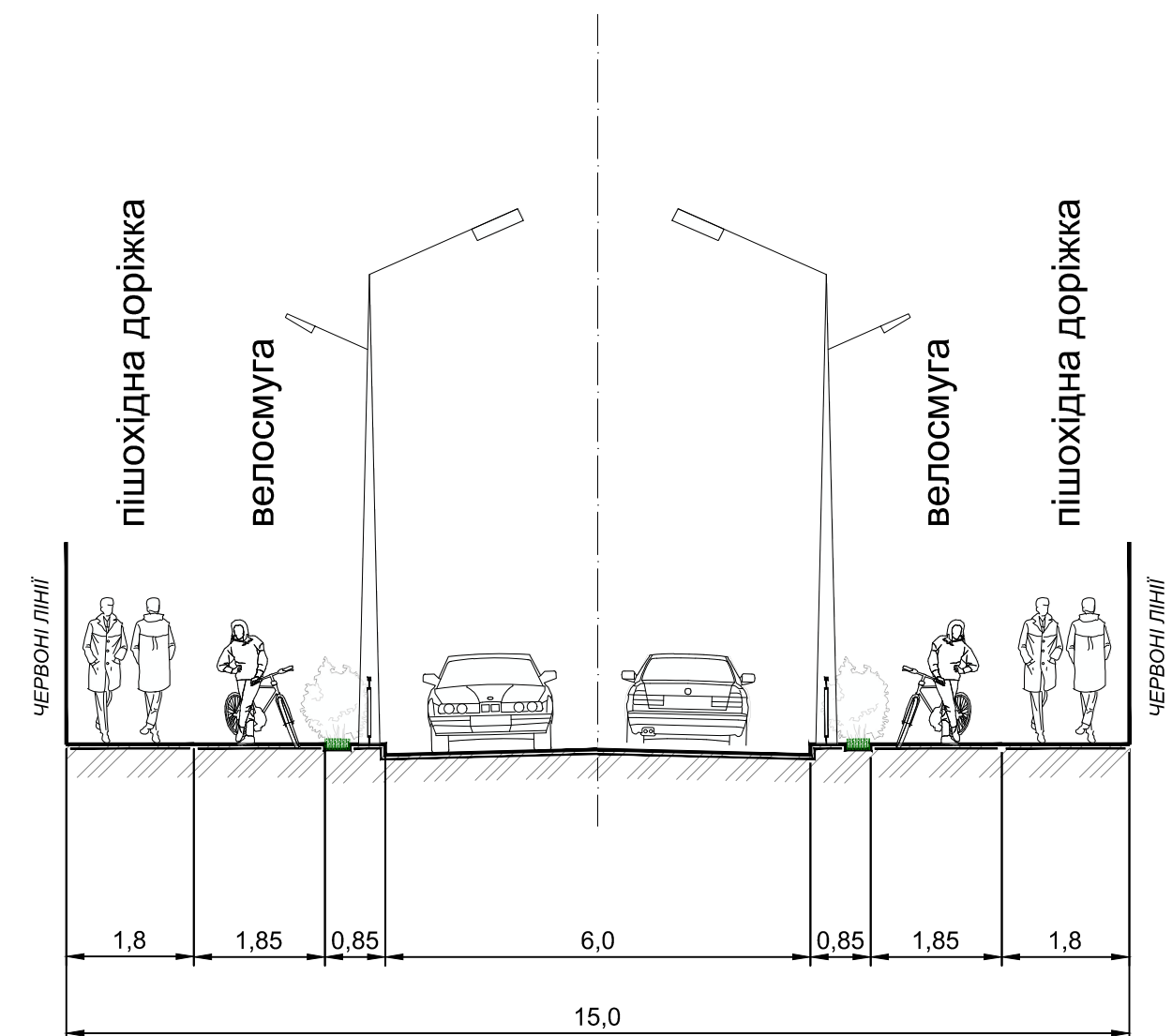
ПРОФІЛЬ 1 - 1 вул. АСКАНІЯ
