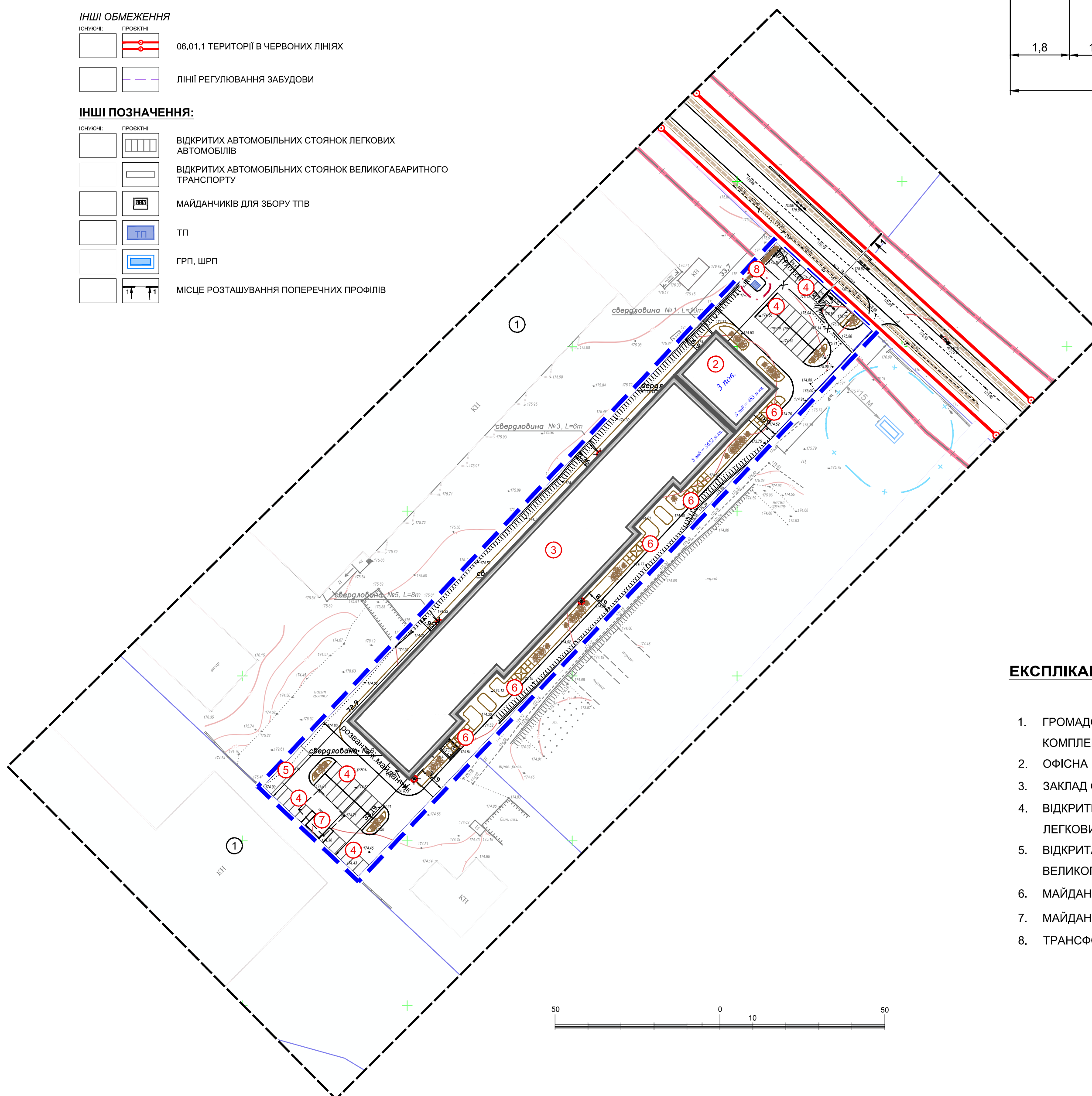
СХЕМА РОЗТАШУВАННЯ ПОПЕРЕЧНИХ ПРОФІЛІВ М 1:1000
