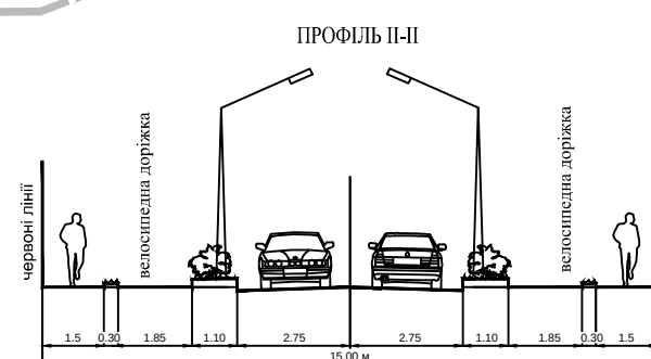
ПОПЕРЕЧНІ ПРОФІЛІ ВУЛИЦЬ М 1:200:
